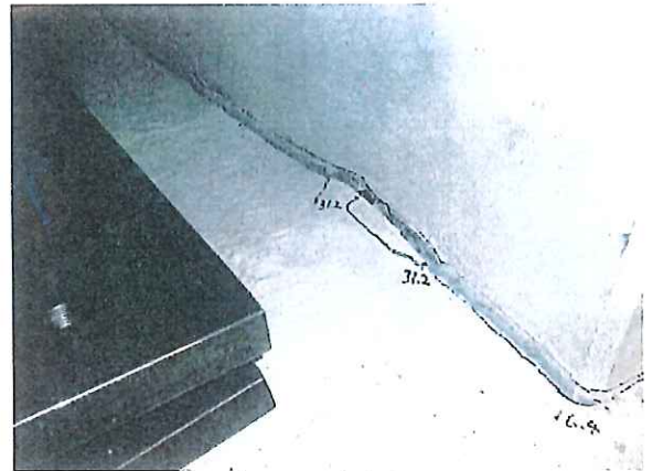
写真2 破壊状況 試験体記号：AW12-1 Pmax=33.3 kN ・補強筋の引き抜け
