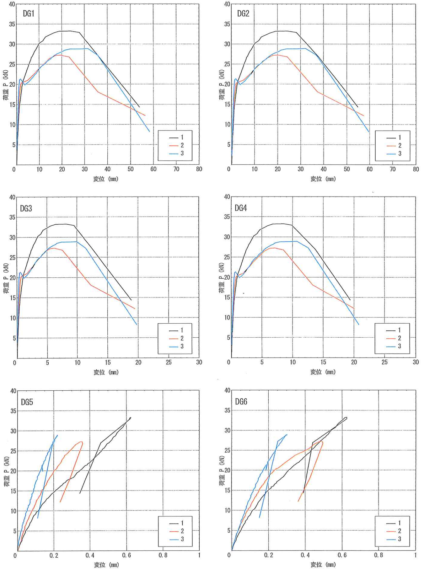
図4 荷重—各部の変位曲線
