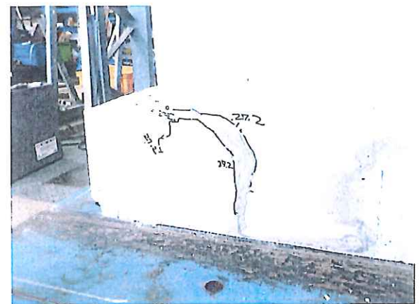
写真6 破壊状況 試験体記号：AW12-2 Pmax=27.2 kN ・擁壁隅角部で底板の割れ
