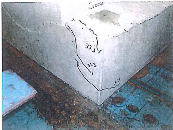
写真3 破壊状況 試験体記号：AW12-1 Pmax=33.3 kN ・擁壁隅角部で底板の割れ
