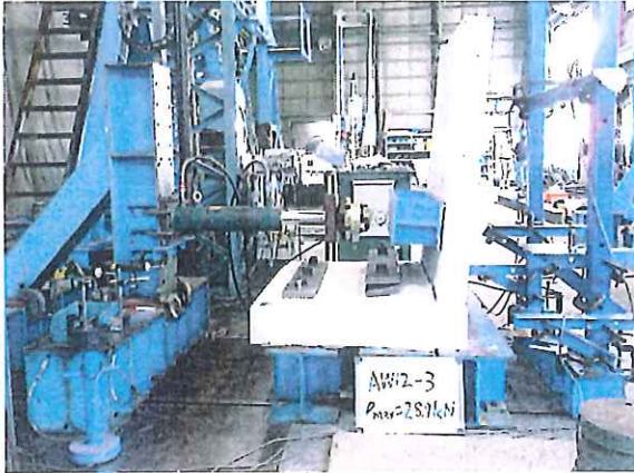
写真7 破壊状況 試験体記号：AW12-3 P_{max}=28.9\text{ kN} ・全景
