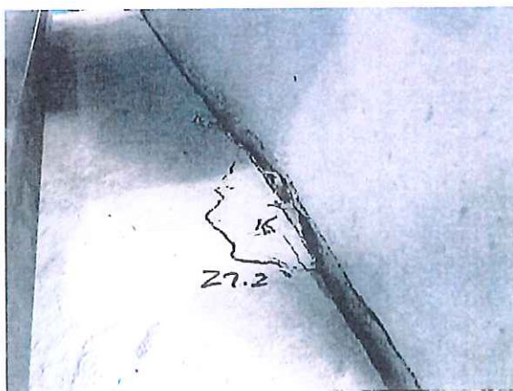
写真5 破壊状況 試験体記号：AW12-2 Pmax=27.2 kN ・補強筋の引き抜け
