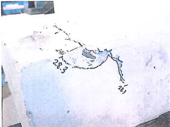
写真9 破壊状況 試験体記号：AW12-3 P_{max}=28.9\text{ kN} ・擁壁隅角部で底板の割れ
