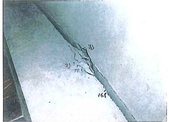
写真8 破壊状況 試験体記号：AW12-3 P_{max}=28.9\text{ kN} ・補強筋の引き抜け
