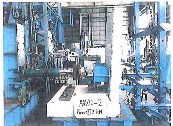
写真4 破壊状況 試験体記号：AW12-2 Pmax=27.2 kN ・全景
